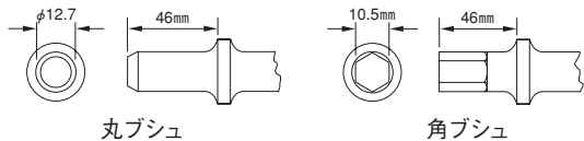
AA-00チゼル差込寸法(カラータイプ)
