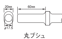
AA&PBチゼル差込寸法
